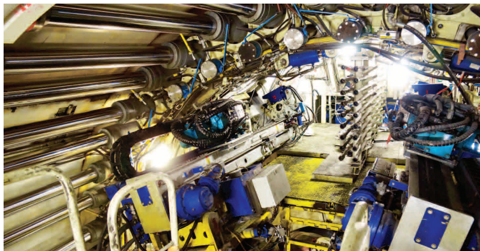
Le tunnelier est équipé de deux foreuses à l'avancement, permettant la réalisation de sondages destructifs et carottages ▲
